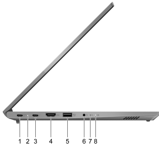
Rysunek 4. Widok z lewej strony—ThinkBook 14 G2 ITL i ThinkBook 15 G2 ITL
