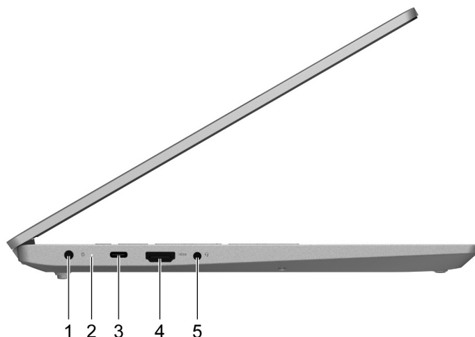
Rysunek 6. IdeaPad 5 (15", 05) i IdeaPad Slim 5 (15", 05) - widok z lewej strony
