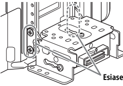
Esiasennetut ruuvit
