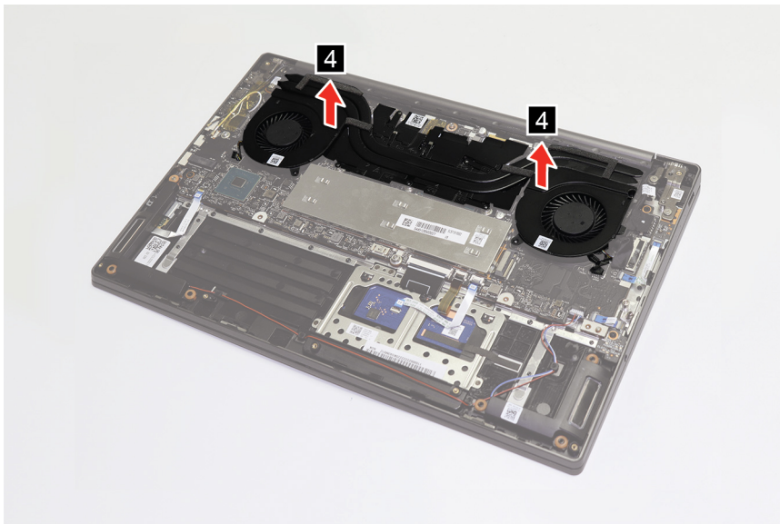
Figure 12. Remove the thermal module
