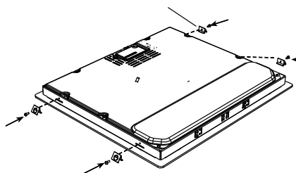
Monteringsfäste bänkskiva
