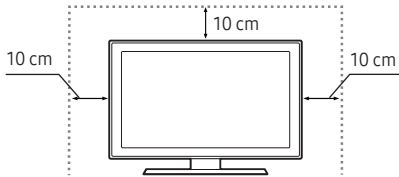
Felszerelés állványra
