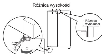
Lewa śruba regulacji wysokości
