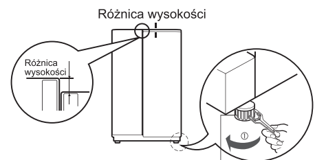
Prawa śruba regulacji wysokości
